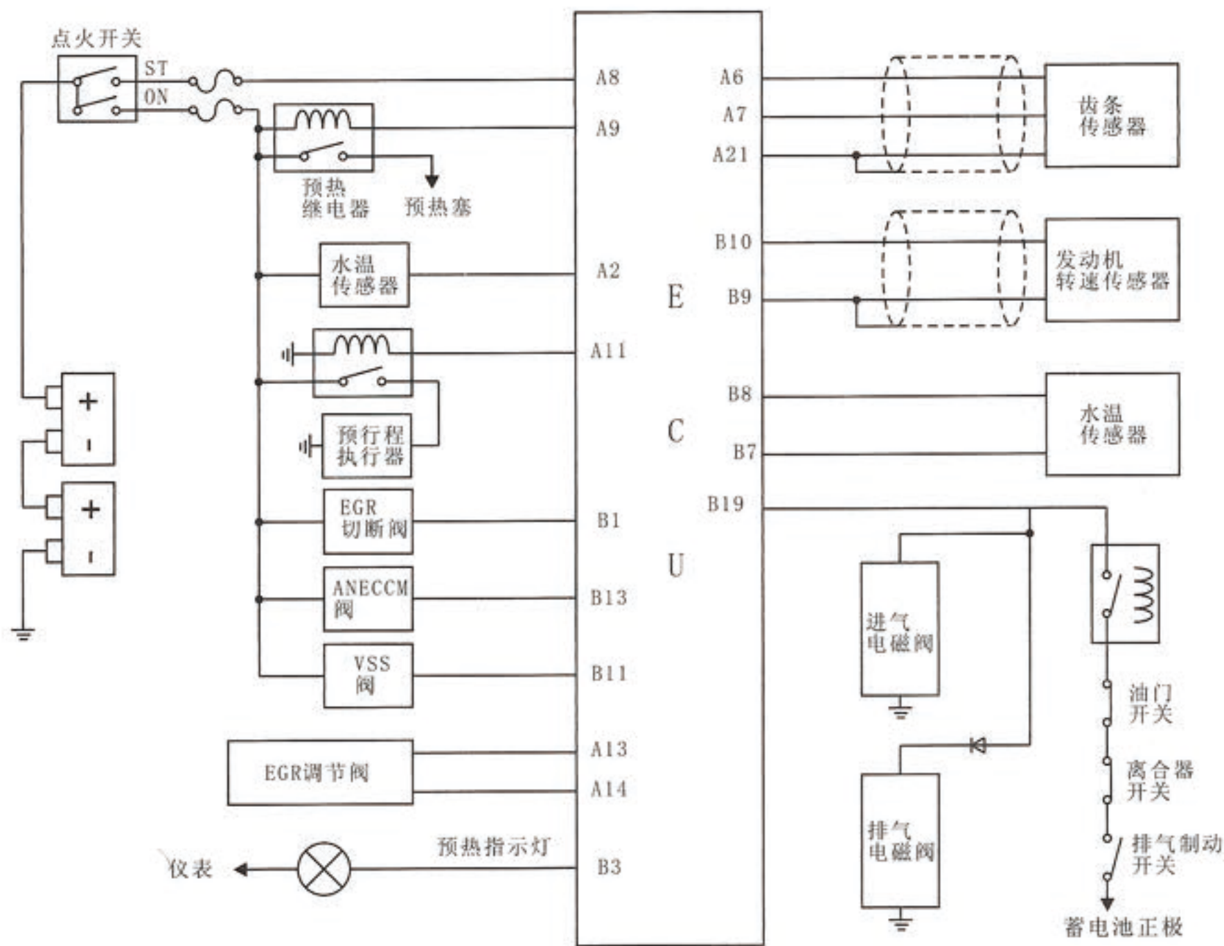
五十铃4HE1发动机ECU端子定义
