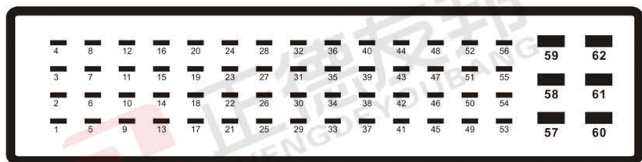
B 端口(白色)
